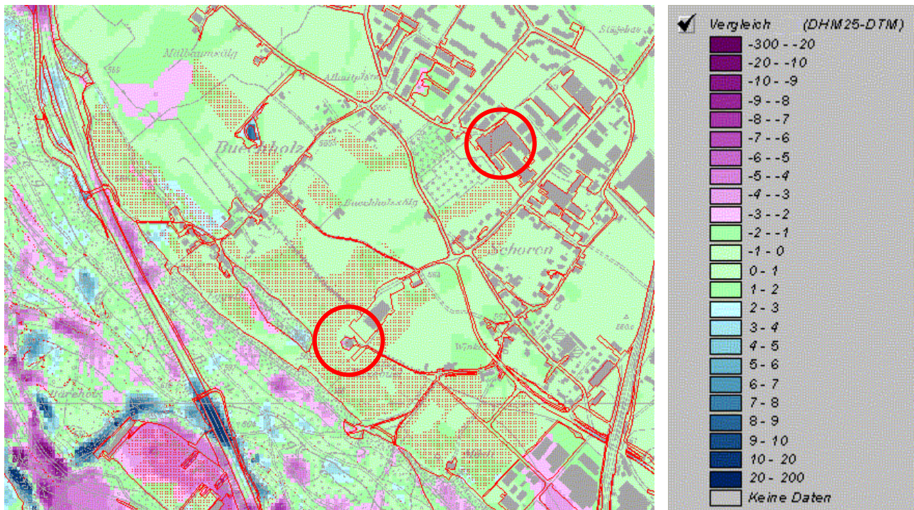
Abbildung 7: Differenzflächen zwischen 2 Terrainmodellen (Differenzklassen in [m]).
